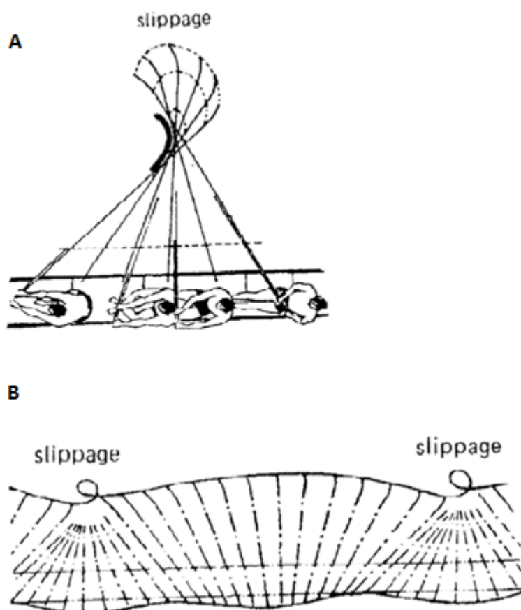
Figur 1.3.4 A og B: Figurerne viser hvordan åren næsten står stille i vandet, mens båden og roeren flytter sig i fremdriftsretningen. (Kilde: Rowing, Dr. Ernst Herberger, et. al.)
