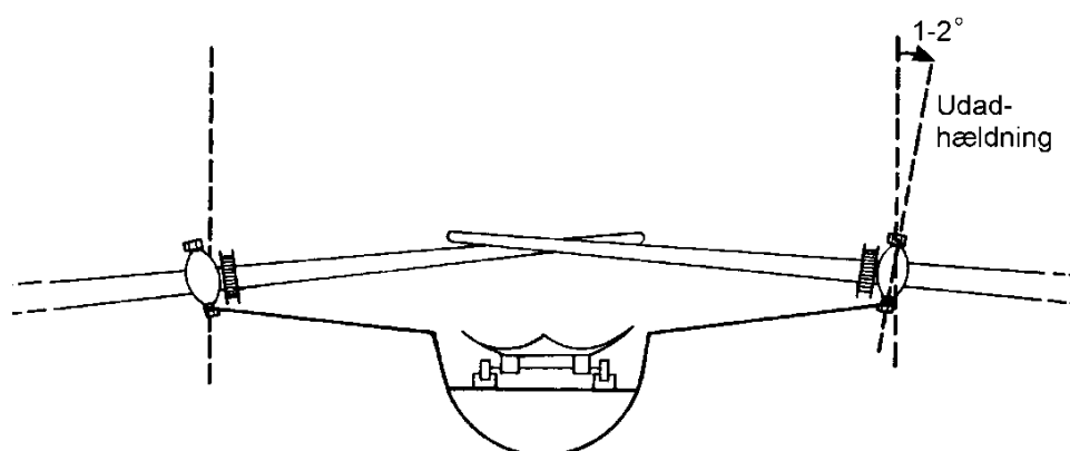
Figur 3.5.1: Figuren illustrerer udafhældningen på svirvlen på en singlesculler (Kilde: Rowing – The Skills of the Game, Rosie Mayglothling, 1990, let tilrettet).
