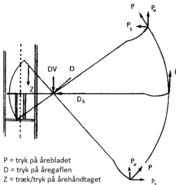
Figur 1.3.1: Årens kraftoverførelse med omdrejning om svirvlen set i tre positioner. (Kilde: Rowing. Dr. Erns Herberger et. al.)
