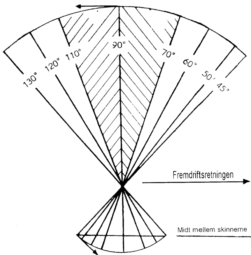
Figur 1.3.2: Det mest effektive trækomsråde er mellem 70° og 110°, også kaldet kernetaget, og er markeret med skravering (Kilde: Rowing: Dr. Ernst Herberger et. al.).
